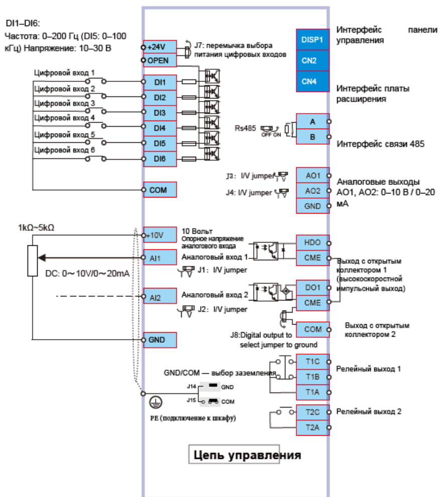
Рисунок 2 – Схема подключения
